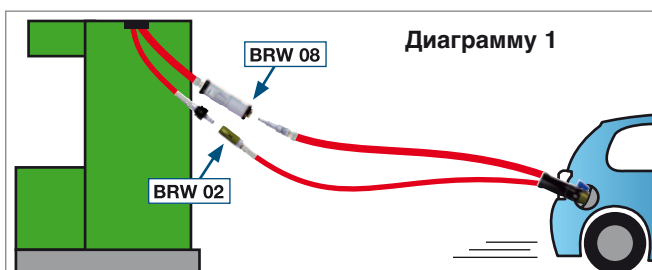
Быстрая заправка легковых или грузовых автомобилей: BRW 08 на линии заправки и BRW 02 на линии сброса.
