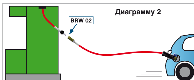
Медленная заправка только легковых автомобилей: BRW 02 только на линии заправки (вентиляционная линия отсутствует).
